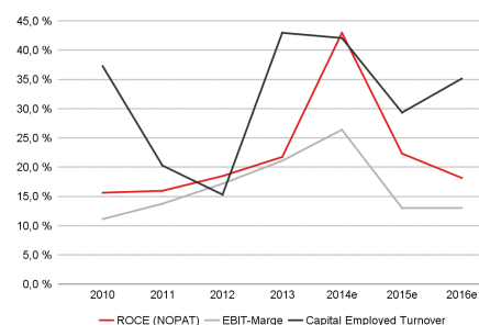
ROCE Development
